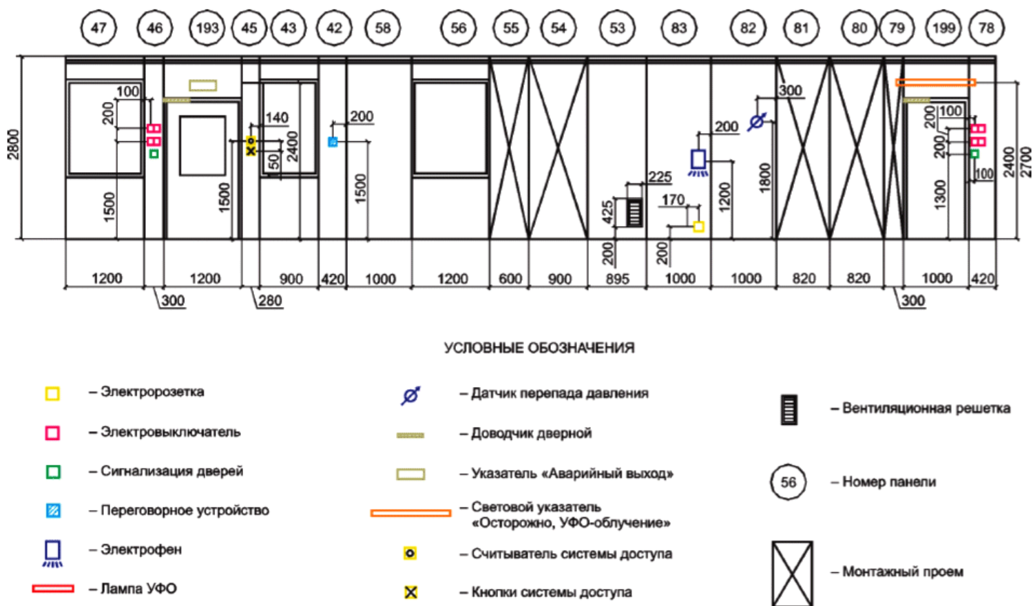
Рисунок 1 - Развертка стены чистого помещения
